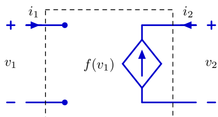
VCCS i_1 = 0 i_2 = -f(v_1)
