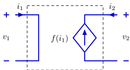
CCCS v_1 = 0 i_2 = -f(i_1)
