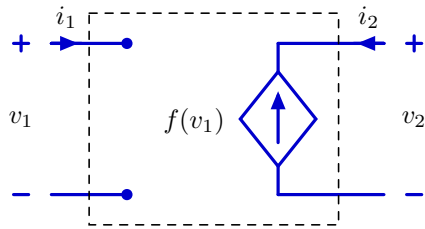
VCCS i_1 = 0 i_2 = -f(v_1)
